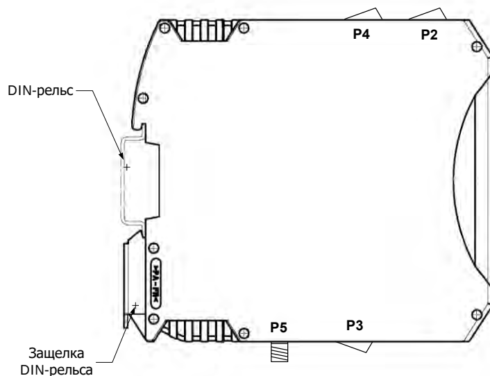
Рисунок 2. Источник первичный точного времени RTNTP-1A. Вид сбоку
